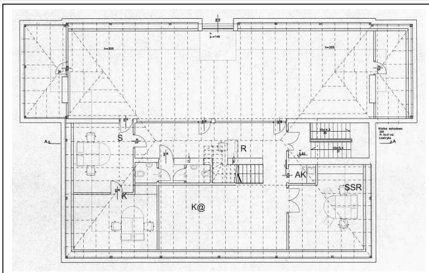
Rzut poziomy poddasza
