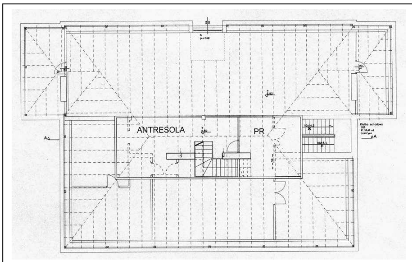
Rzut poziomy antresoli
